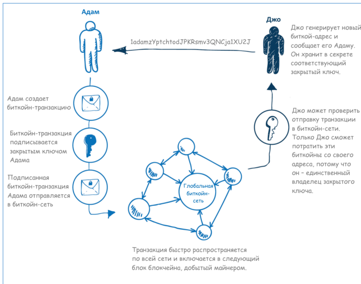
Рис. 1. Адам посылает Джо биткойны через биткойн-сеть
