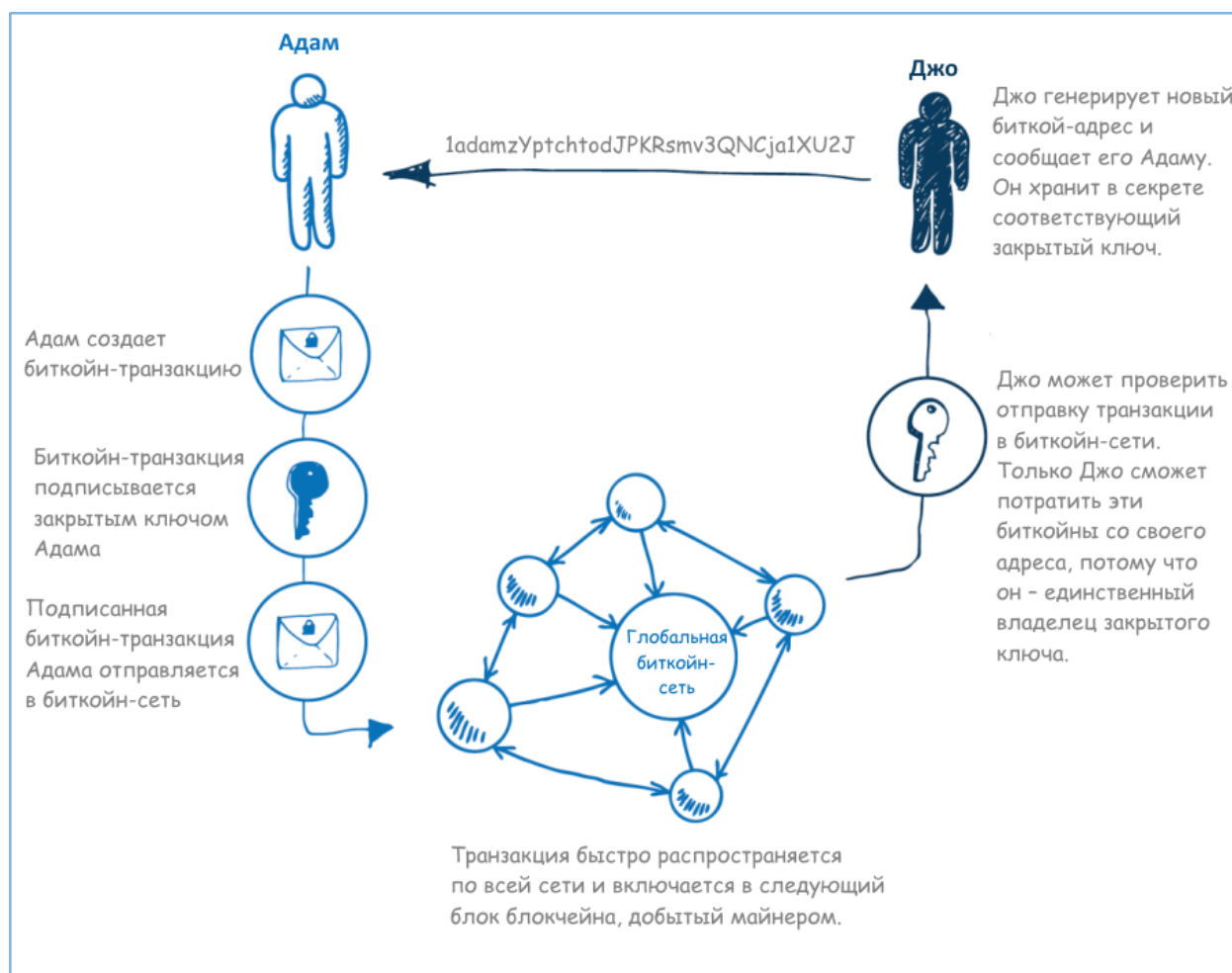
Рис. 3. Адам посылает Джо биткойны через биткойн-сеть
