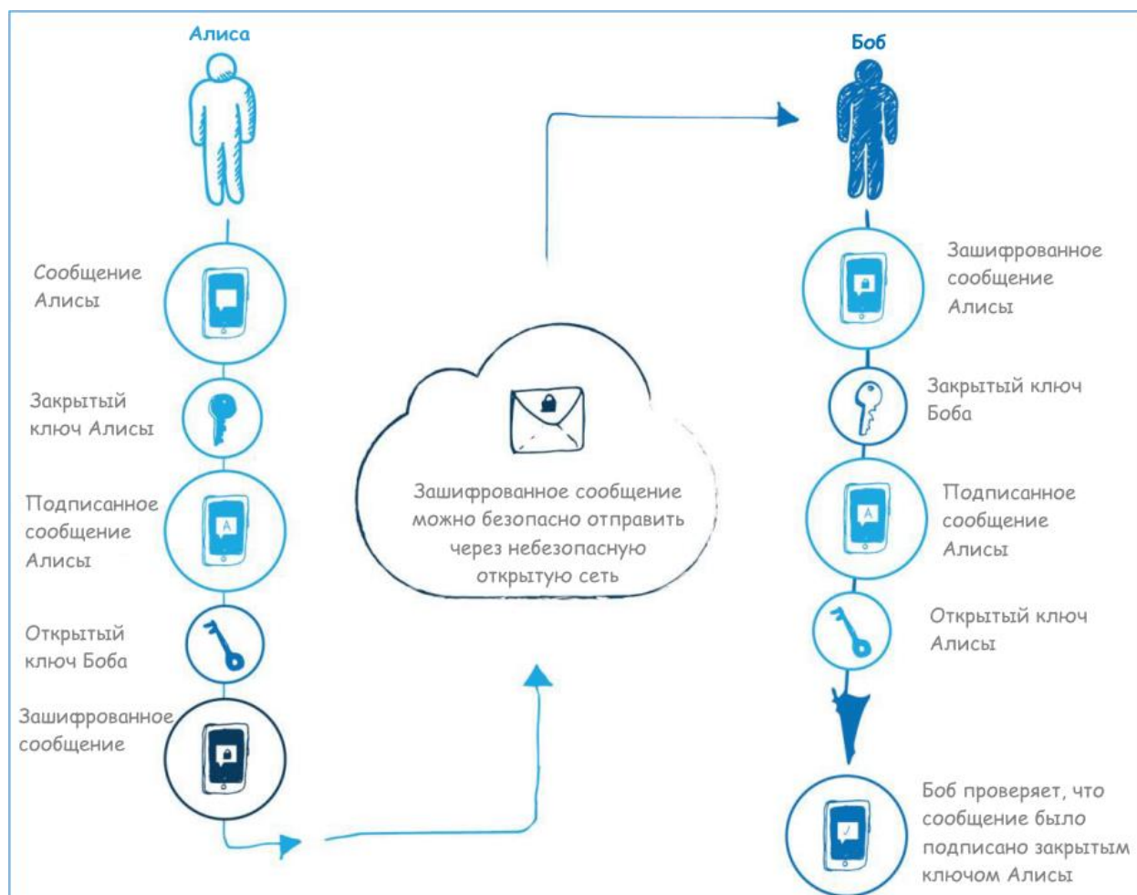
Рис. 2. Асимметричное шифрование. Алиса посылает подписанное зашифрованное сообщение Бобу.
